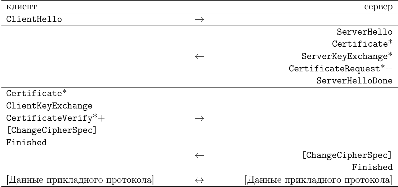
Рисунок 1 — Полный обмен сообщениями протокола Handshake
