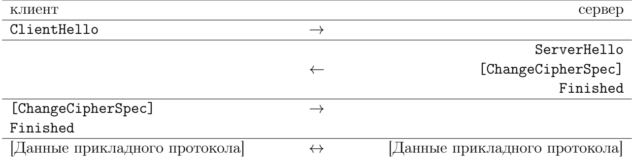
Рисунок 2 — Сокращенный обмен сообщениями протокола Handshake
